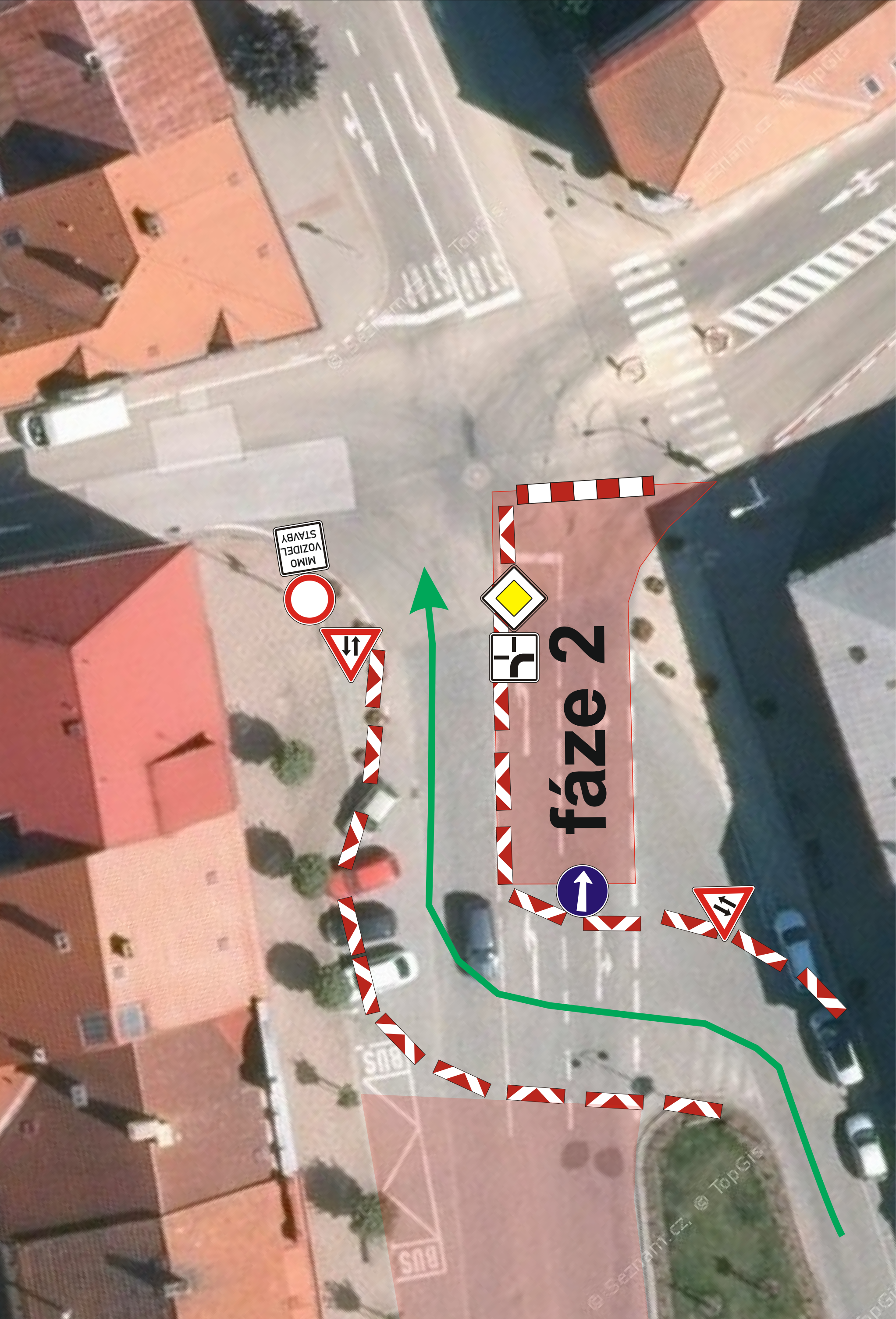
Dopravně inženýrské opatření v průběhu prací na krytu vozovky v místě výjezdu z nám. Jiřího z Poděbrad na ul. Riegrova - fáze 2
